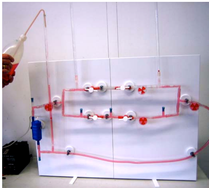
Abb. 6: ... dann durch das untere Manometerrohr
