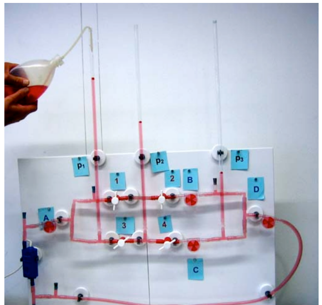
Abb. 12: Der absolute Druck steigt durch das Hinzufügen von Wasser, alle Druckdifferenzen bleiben jedoch gleich.
