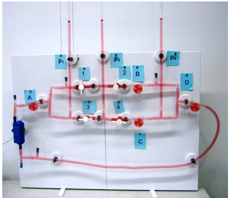
Abb. 2: Wasserstromkreis mit eingebauten Manometerröhren
