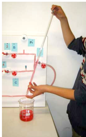
Abb. 8: Wasser wurde angesaugt und dann das Rohr oben verschlossen.
