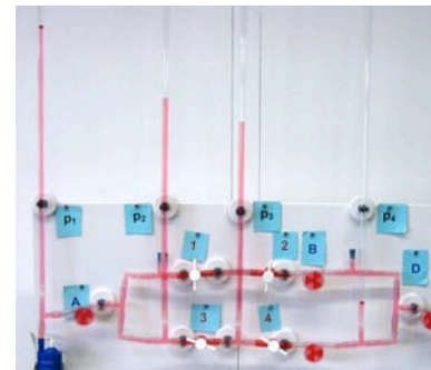
Abb. 11: Der Druckverlauf längs des Stromkreises wird sichtbar.
