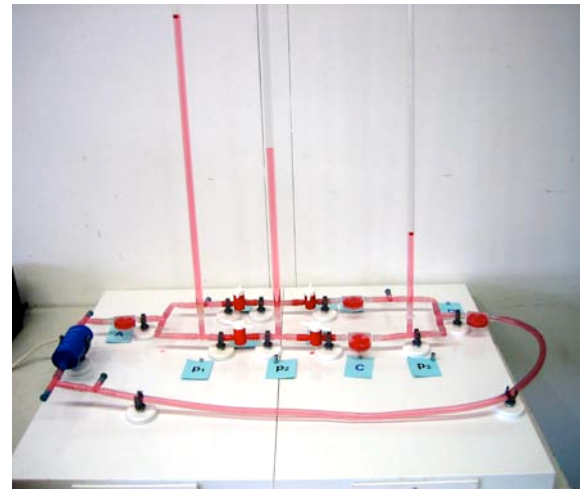
Abb. 13: Wasserstromkreis vertikal betrieben.
