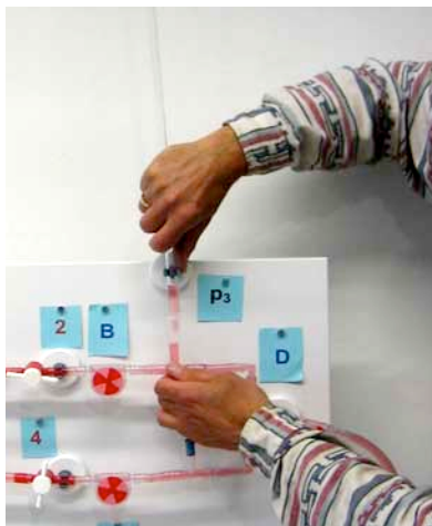
Abb. 7: Das Monometerrohr kann Im gefüllten Stromkreis eingebaut werden
